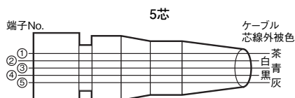
結線図
