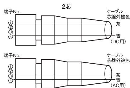
結線図
