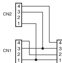
配線図
