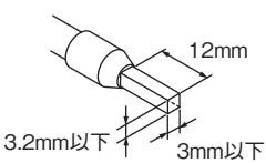
フェルル端子の加工寸法
