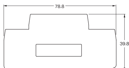
形XW5E-P2.5-1.1-2
