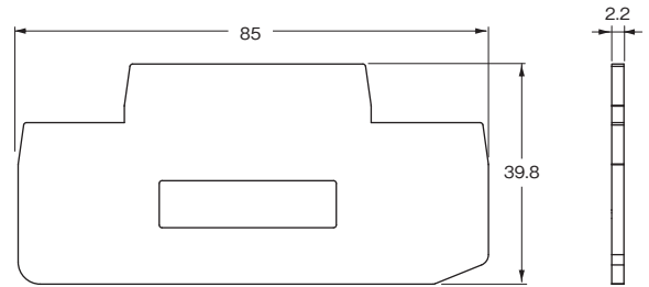
形XW5E-P4.0-1.1-2
