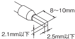
フェルル端子の加工寸法
