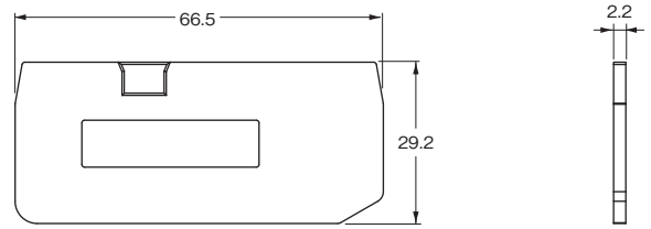
形XW5E-P4.0-1.1-2
