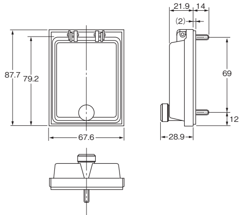
形Y92A-48N (48□用)
