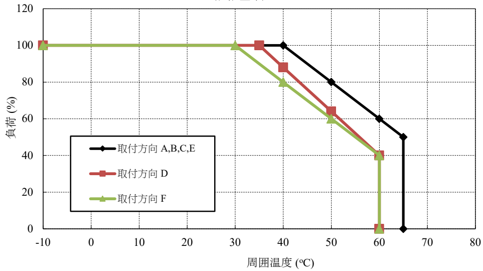
負荷 対 周囲温度 (自然空冷)
