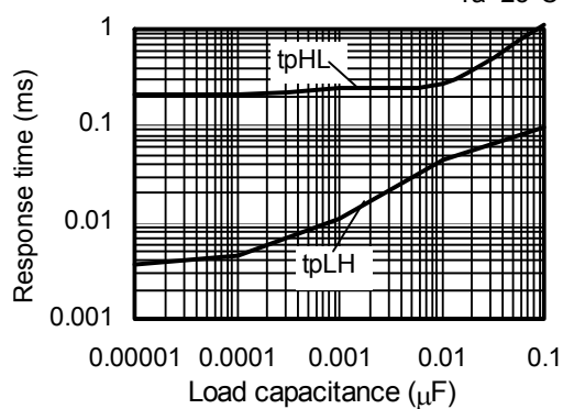
S-80914CL T_a=25^\circ\text{C}
