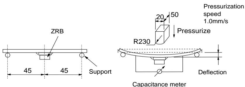
Fig.2 (in:mm)
