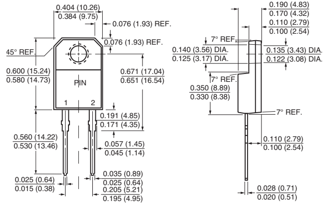
ITO-220AC
