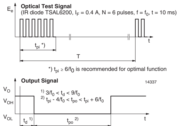
Fig. 1 - Output Function
